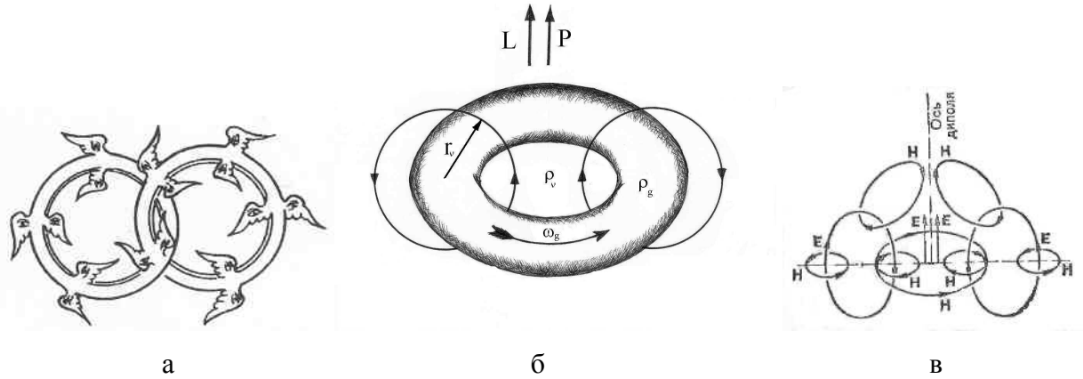
Рис 2. Вихревая модель ЭФ (б), а) – ее мифологический образ (престолы) и в) – ЕН-вихри диполя.
