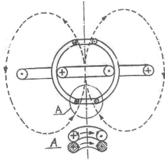
Схема внутренней структуры электрона. Пунктирные линии v -вихри, заштрихованы левые вихри.
