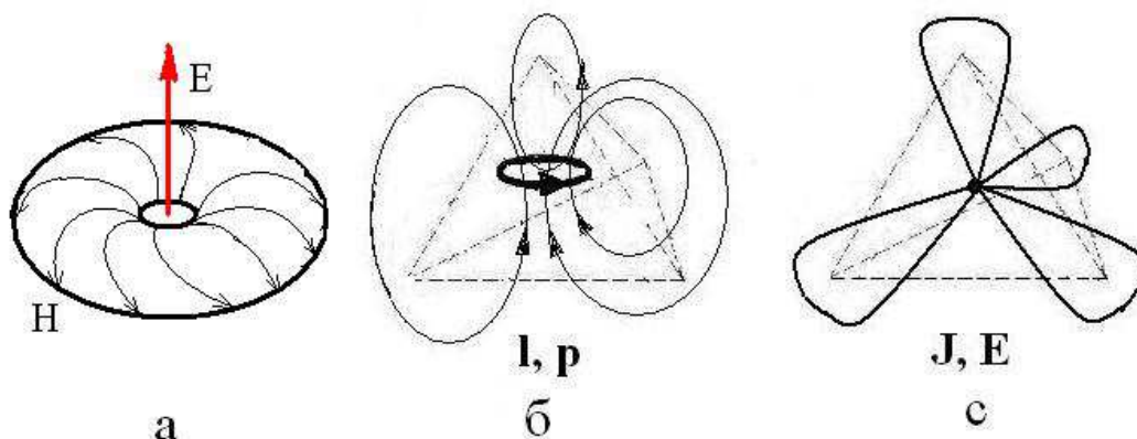
Рис. 1. Модели хирального ЭМ-вихря [10] (а), хирального кванта с моментом импульса – l и импульсом – p (б) и схема sp^3 -гибридизации валентных электронов атома. J – ядерный спин, E , H – напряженности электрического и магнитного поля.
