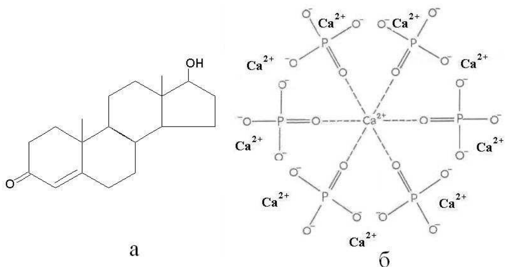
Рис. 4. Структуры полового гормона тестостерона (а) и молекулярной основы костного материала – кристалла гидроксиапатита (б).
