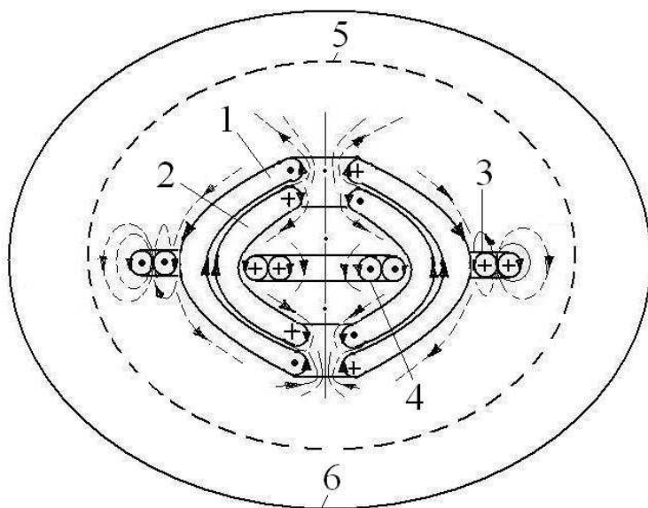
Рис 2. Модель структуры остова («ядра») Солнца.
