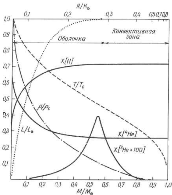
Рис 1. Эмпирические и расчетные данные по структуре Солнца [9].
