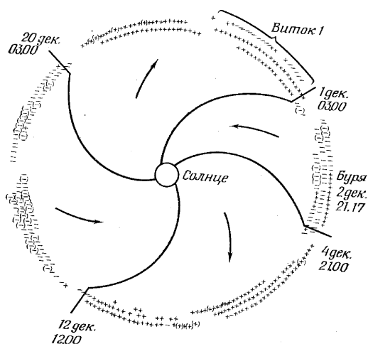
Рис 8. Четыре сектора магнитного поля Солнца. Прообразы свастики и Креста Христова.
