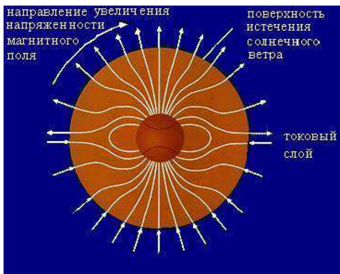
Рис 4. Магнитное поле Солнца
