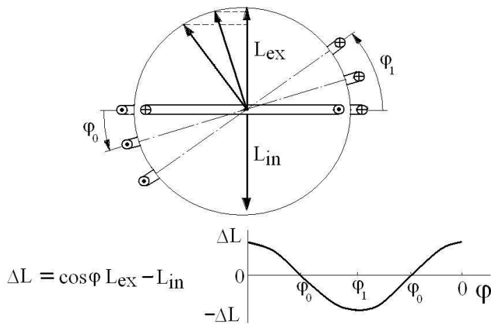
Рис 3. Схема гармонических колебаний внешней орбиты Солнца (момент импульса L_{ex} ) относительно неподвижной внутренней орбиты ( L_{in} ). Период колебаний – изменения угла от 0 до \varphi_1 составляет ~22 года. При значении угла \varphi_0 происходит переполюсовка магнитного поля Солнца. Угол \varphi_0 может быть равен углу наклона оси вращения Солнца к плоскости эклиптики ( 7^\circ 15' ).
