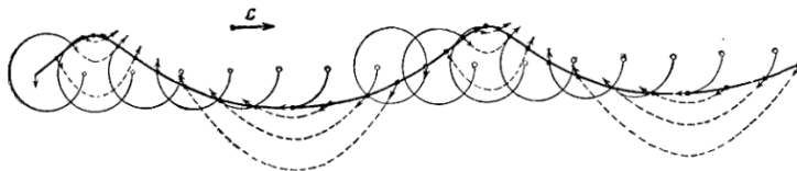
Рис. 437. Связь линий тока и круговых путей в бегущих водяных волнах. Горизонтальный ряд точек показывает частички поверхности воды в состоянии покоя, дуги окружностей — пути, пробегаемые ими по направлению часовой стрелки. Соединив маленькие острия стрелок , мы получаем профиль распространяющейся вправо волны в конце следующего промежутка времени. Круговые траектории вычерчены для каждой второй стрелки.
