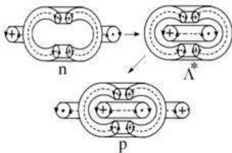
Рис 6. Схема перестройки структуры нейтрона ( n ) в структуру протона ( p ) через промежуточное виртуальное \Lambda^* -состояние нейтрона. Пунктир означает, что субэлементы состоят из m/e -пар.
