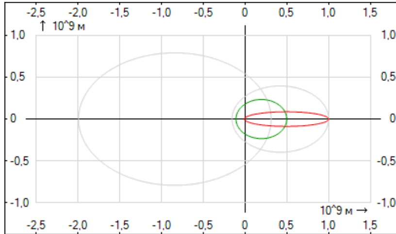
Рис. 7. Траектории тел в системе центра масс по «методу».
