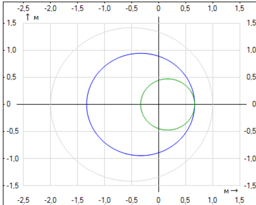
Рис. 6. Траектории тел в системе центра масс.
