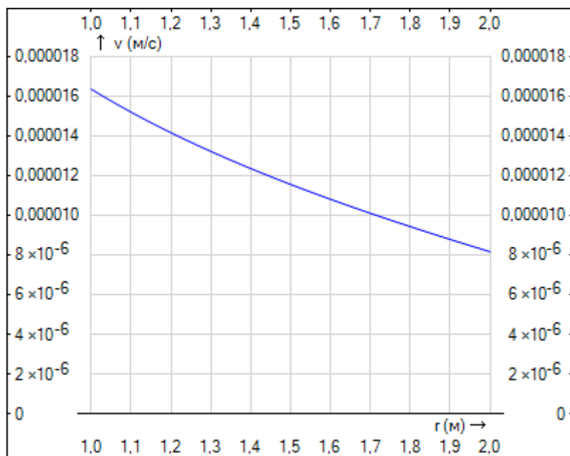
Рис. 2 . Скорость тела в относительной системе отсчёта в интервале [p, a] .
