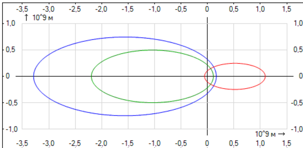
Рис. 9. Траектории при a = 3,3 \cdot 10^9 м.
