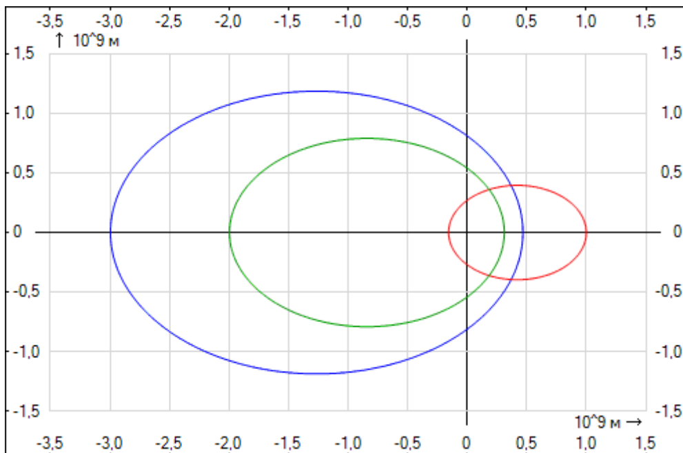
Рис. 8. Траектории тел в обеих системах отсчёта при a = 3,0 \cdot 10^9 м.
