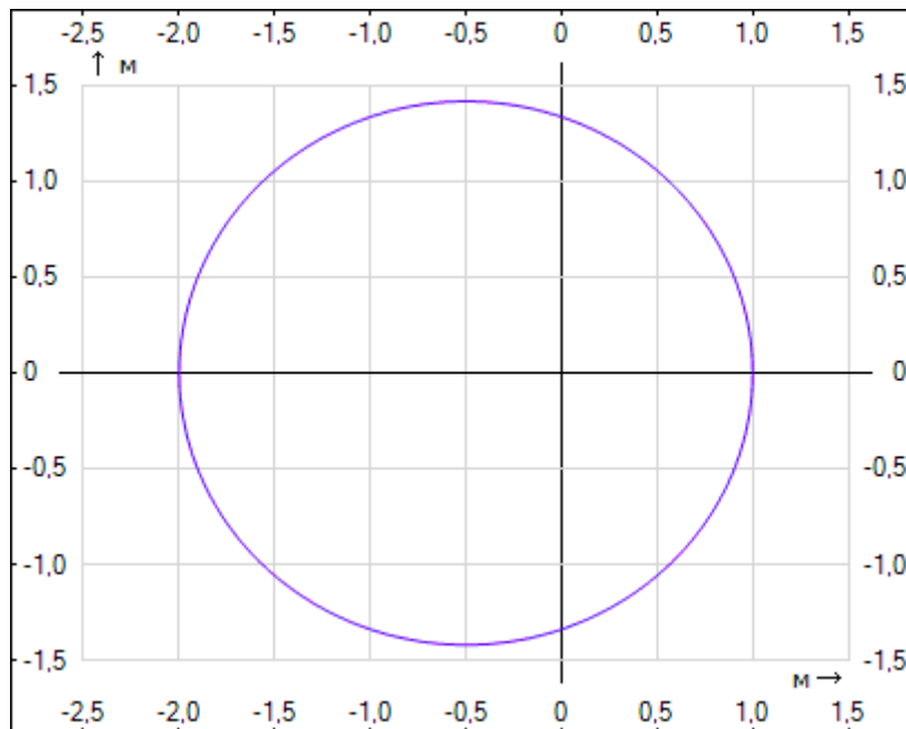
Рис. 5. Траектория тела в относительной системе отсчёта.
