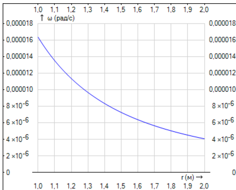
Рис. 1. Угловая скорость тела в интервале [p, a] .
