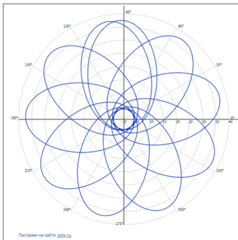
Рис. 10. Орбита спутника чёрной дыры OJ 287. Смещение составляет 39^\circ за (двенадцатилетний) период.
