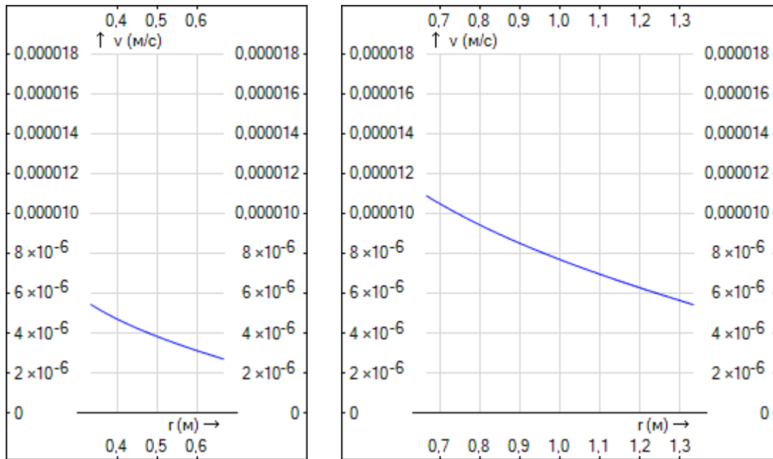
Рис. 3 и 4. Скорости второго и первого тела в системе центра масс, в интервалах [p_2, a_2] и [p_1, a_1] , соответственно.
