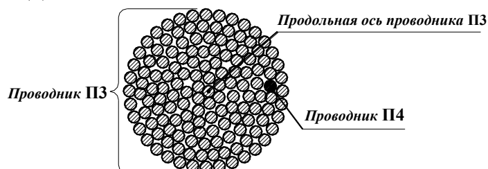
Рис. 5.7. Поперечное сечение многопроволочного проводника
