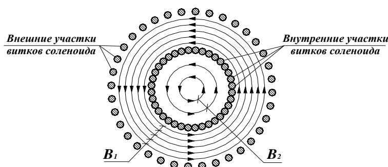
Рис. 5.15. Сечение изогнутого в кольцо соленоида
