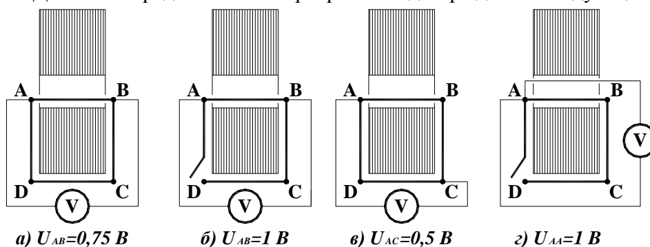
Рис. 5.11. Измерение напряжения на участках витка, находящегося в двух его состояниях
