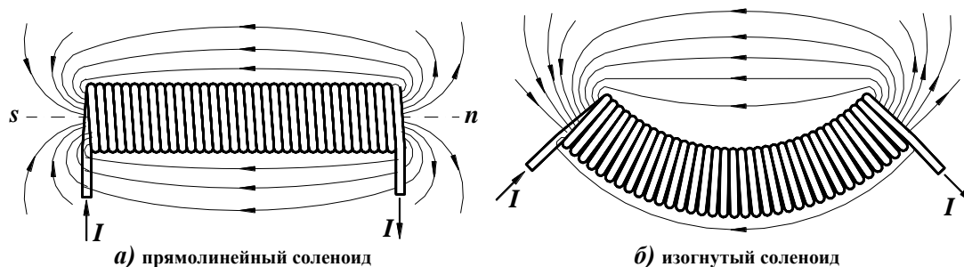
Рис. 5.14. Магнитное поле наведенное током I , текущим в витках соленоида
