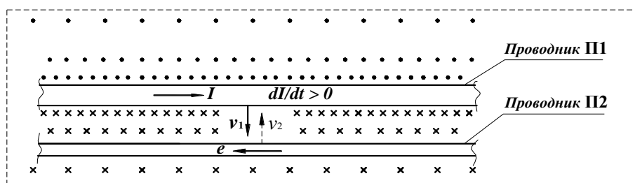
Рис. 5.6. Наведенная в проводнике П2 ЭДС взаимной индукции e
