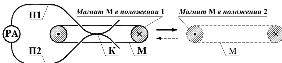
Рис. 5.8. Изменения значения магнитного потока не вызывают наведения ЭДС в замкнутом контуре
