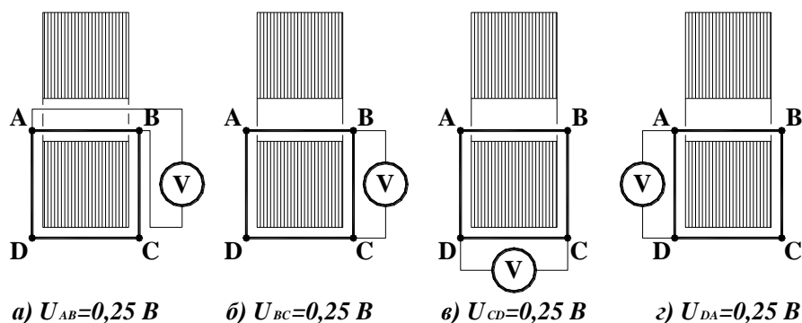
Рис. 5.10. Измерение напряжения на участках короткозамкнутого витка
