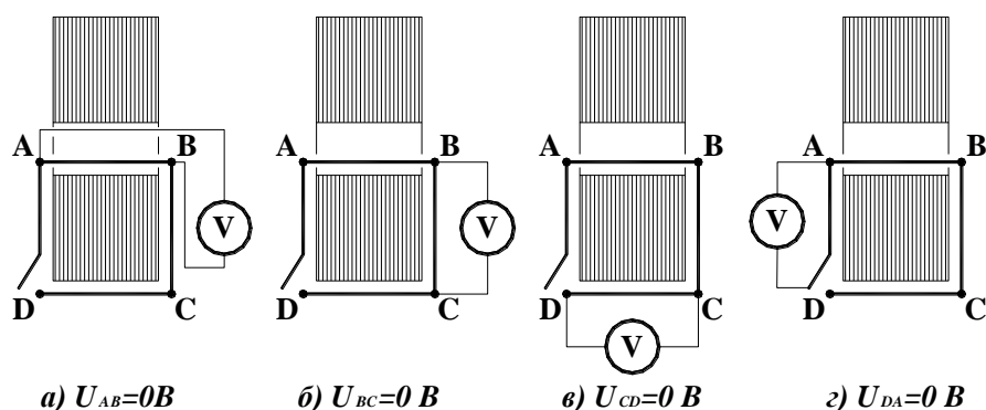
Рис. 5.12. Измерение напряжения на участках разомкнутого витка
