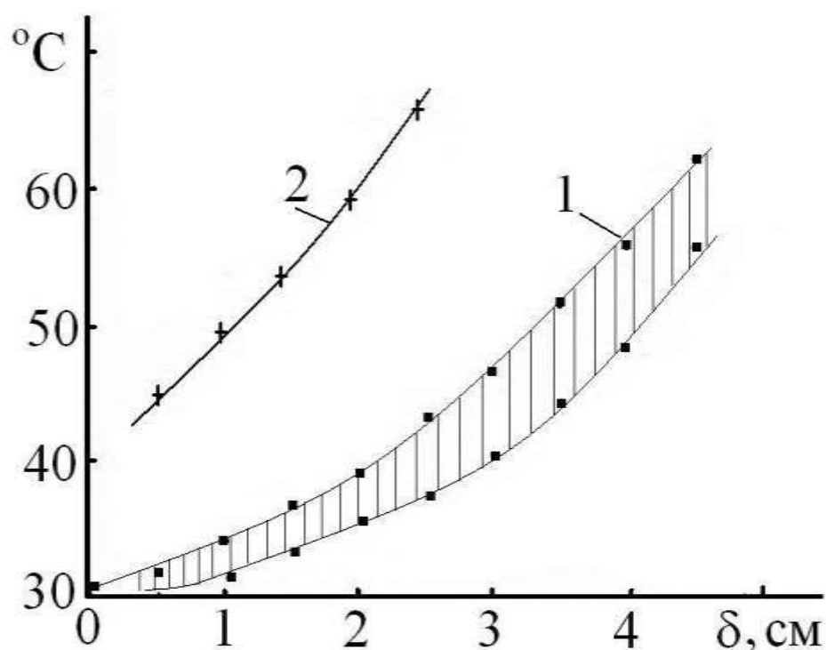
Рис 2. Скорость нарастания температуры вдыхаемого курильщиком дыма в зависимости от длины ( \delta ) выкуренной сигареты (1) и папиросы (2).
