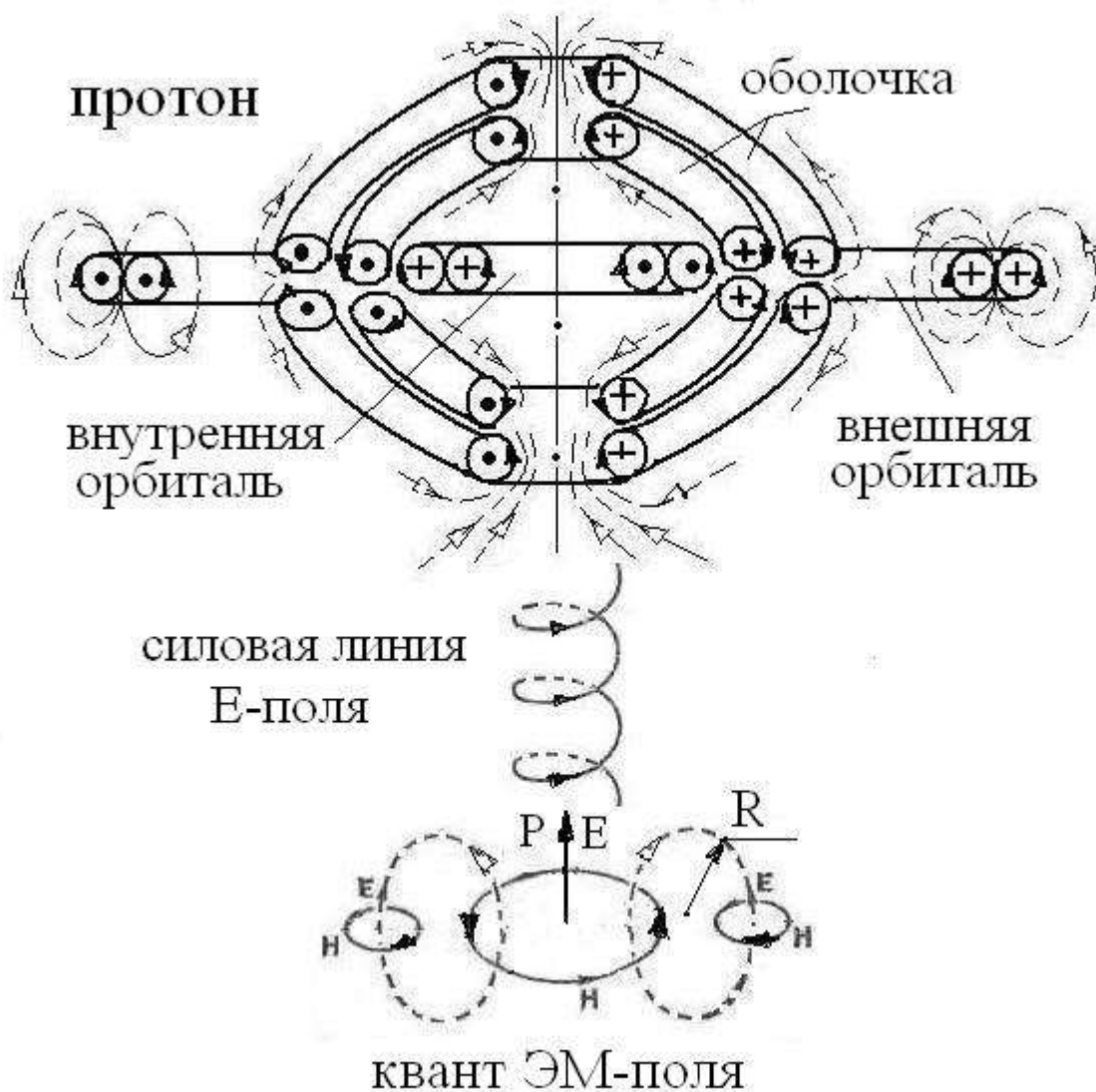
Рис 1. Схема акта поглощения протоном правоспирального кванта ЭМ-поля (ЭМ-энергоформы). Сплошные линии относятся к потокам g -вихрей, а пунктирные - v -вихрей духа. Кольцевые токи v -вихрей вращаются против часовой стрелки и одновременно движутся поступательно. Цуг ЭМ-энергоформ соответствует спирали силовой линии электрического поля.
