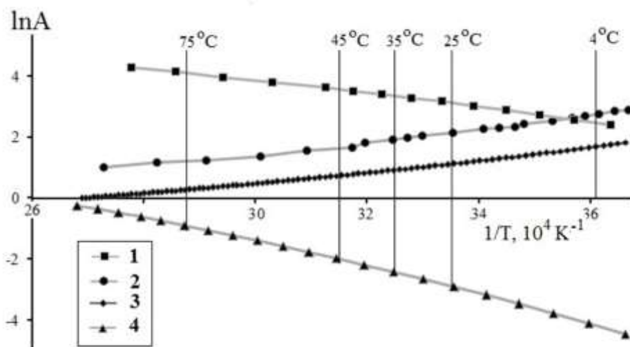
Рис 1. Анаморфозы аппроксимаций температурных зависимостей свойств воды (A): коэффициента самодиффузии (D) – 1; времени диэлектрической релаксации ( \tau ) – 2; динамической вязкости ( \eta ) – 3; электропроводности ( \lambda ) – 4.
