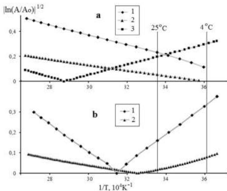
Рис. 2. Анаморфозы аппроксимаций температурных зависимостей свойств воды ( A ): поверхностного натяжения ( \sigma ) – 1а; плотности ( \rho ) – 2а; скорости звука ( v ) – 3а; сжимаемости ( \gamma ) – 1б; изобарной теплоемкости ( C_p ) – 2б. A_0 – значение A в T_{cp} или в T_{\infty} .
