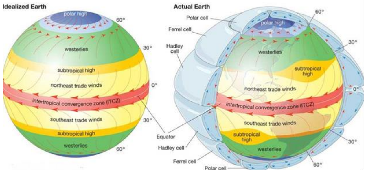
Рис.1 Пояса атмосферного давления.
