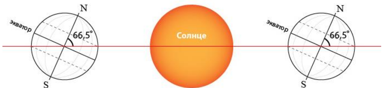
Рис.2 Наклон земной оси к плоскости орбиты.
